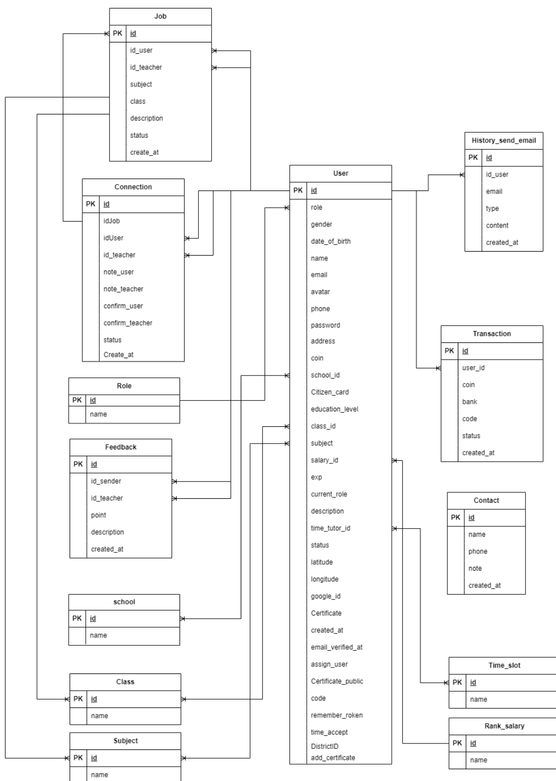
Hình 3.9.1: Mô hình quan hệ thực thể (ERD)
