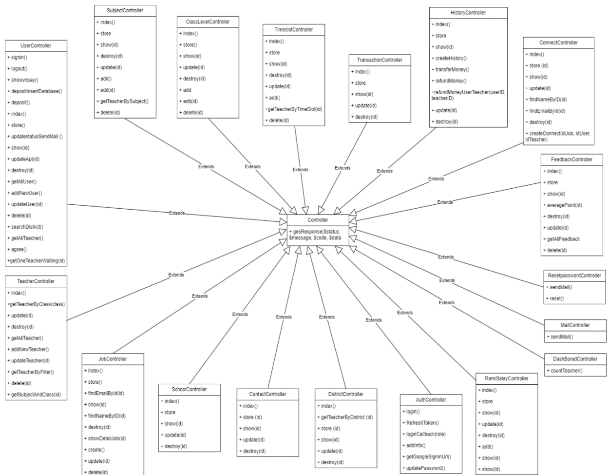
Hình 3.8: Sơ đồ Class Diagram Controller
